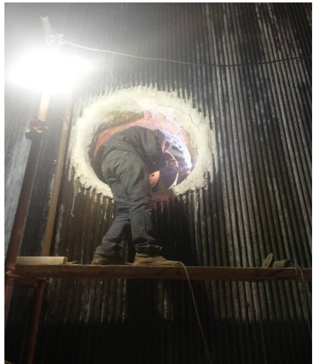
جوشکاری و رفع عیب نازل و دهانه مشعلهای واحد ۳
